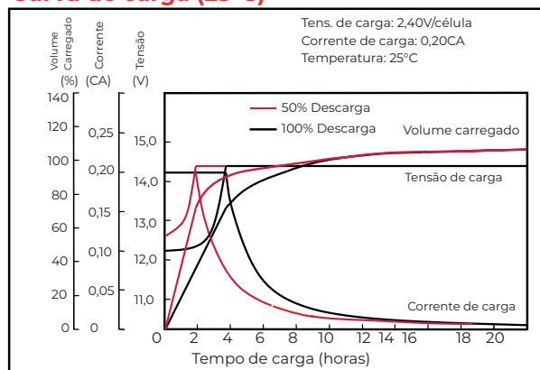
Curva de carga (25°C)
